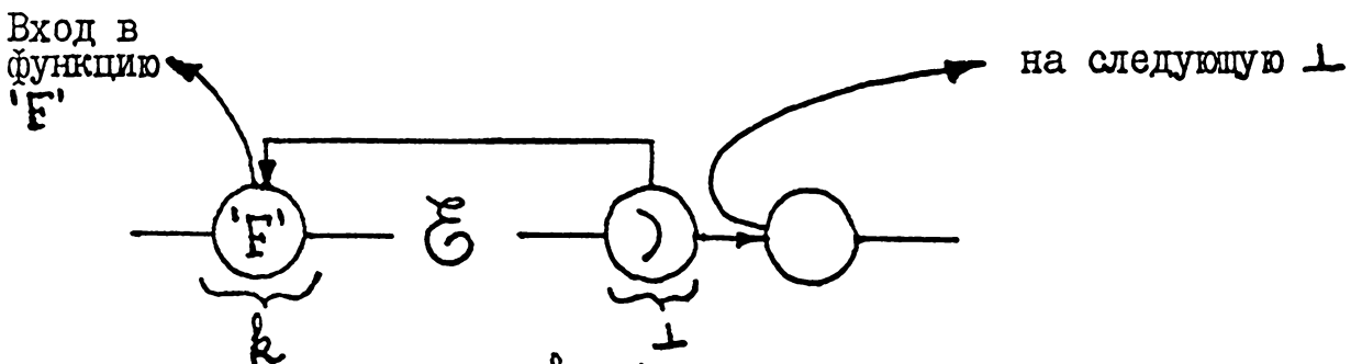
Рис. 3.23. Представление k'F'E⊥ в интерпретаторе языка сборки.
