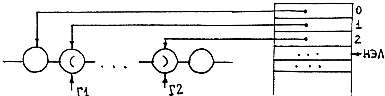
Рис. 3.6. Состояние ТЭ, НЭЛ, \Gamma_1 и \Gamma_2 перед началом шага
