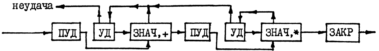
Рис. 3.15. Схема переходов между операторами языка сборки.
