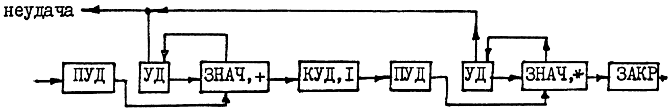
Рис. 3.16. Схема переходов после добавления оператора КУД, I;.
