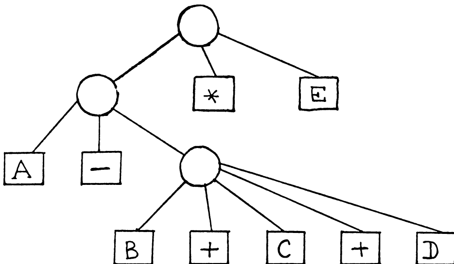
Рис. I.1. Дерево, соответствующее структуре алгебраического выражения (A - (B + C + D)) * E .
