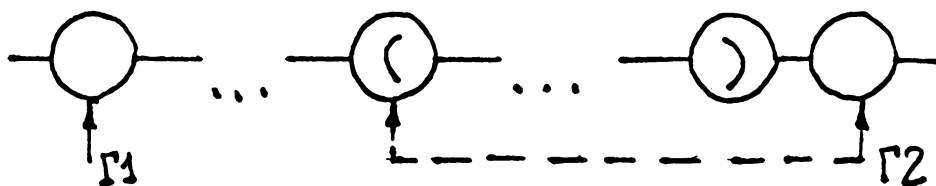
Рис. 3.9. Движение границ при работе оператора СКОБЯ;. .
