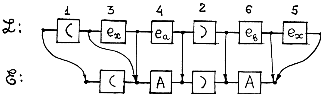
Рис. 2.3. Блок-схема алгоритма отождествления \mathcal{G} как \mathcal{L} .
