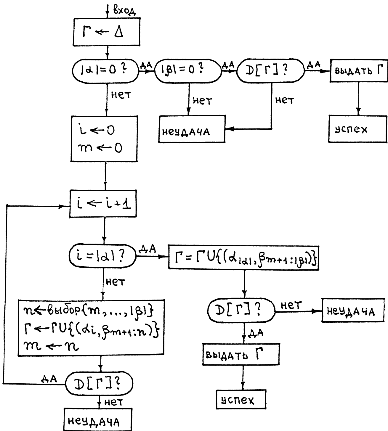
Рис. А .3. Алгоритм отождествления, который учитывает монотонность D[\Gamma]
