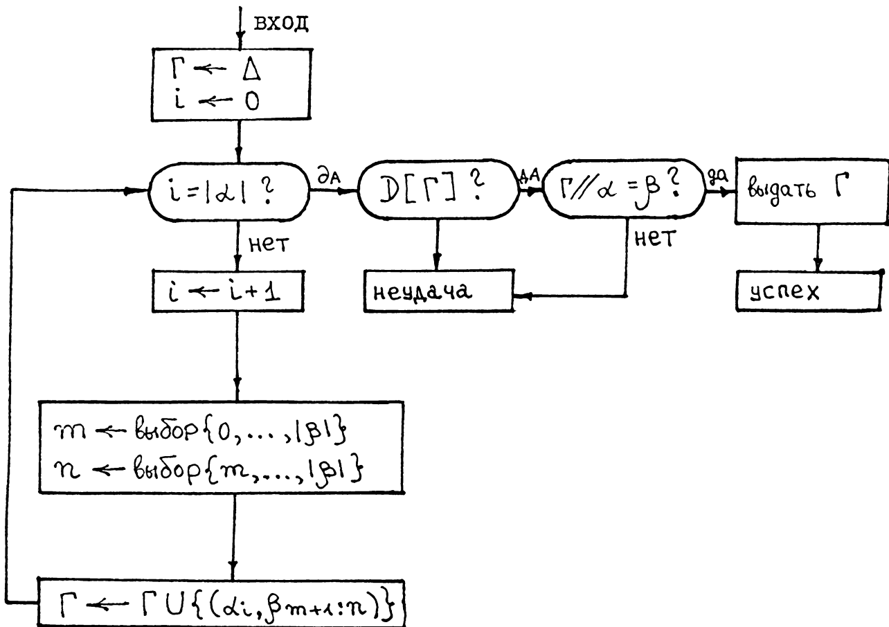
Рис. А.І. Простейший алгоритм отождествления
