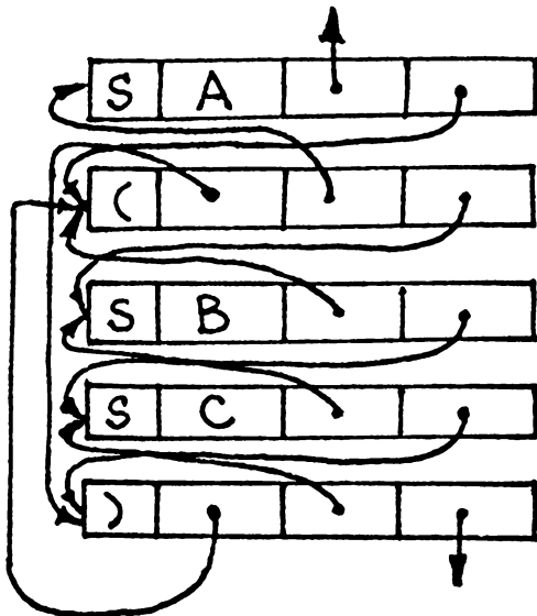
Рис. 3.2. Представление выражения A(BC) в виде списка
