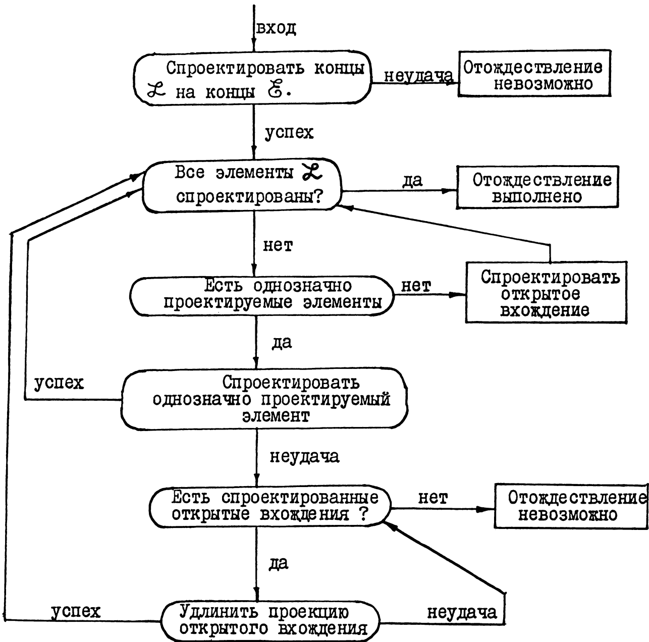
Рис. 2.3. Блок-схема алгоритма отождествления \mathcal{G} как \mathcal{L} .
