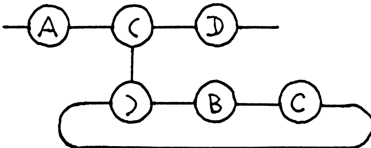
Рис. 3.4. Список, соответствующий выражению A(BC)D, если выбрано другое представление для скобок.
