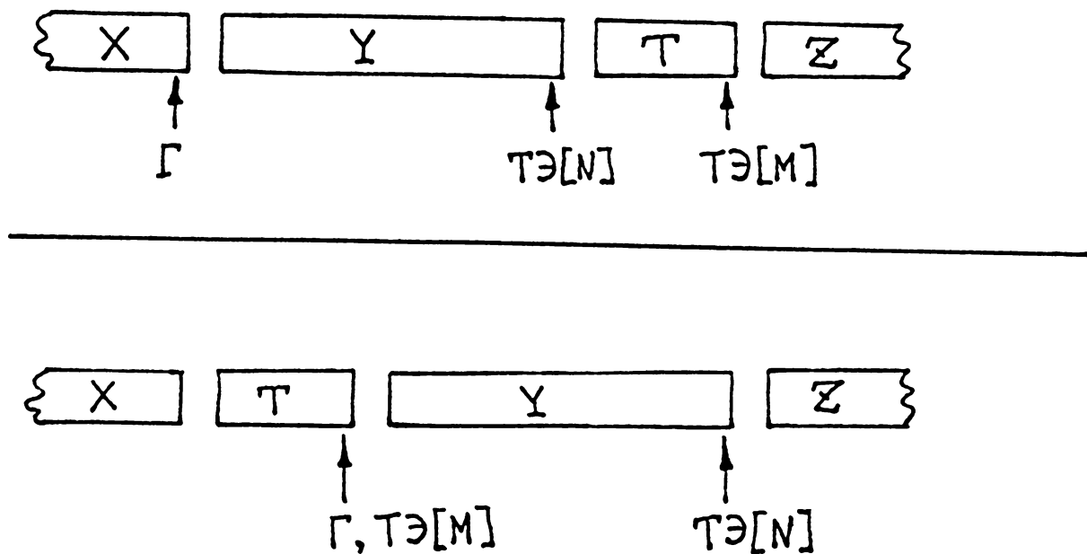
Рис. 3.21. Трансплантация участка T.
