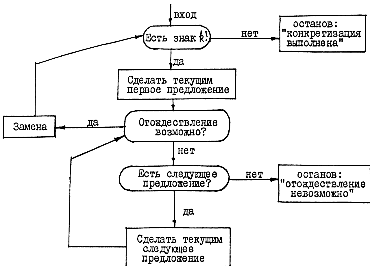
Рис. I.2. Блок-схема рефал-машины.
