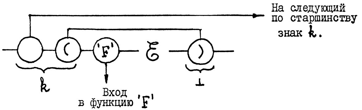
Рис. 3.22. Представление k'F'E⊥ в рефал-интерпретаторе.
