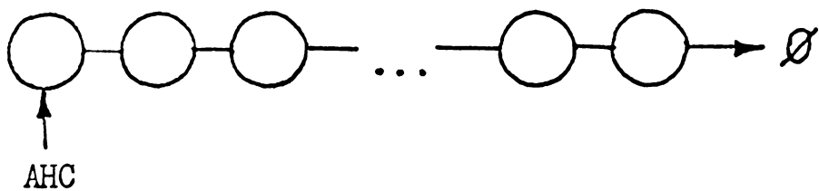
Рис. 3.19. Организация списка свободной памяти.
