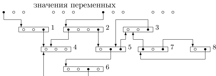
Рис. 1.1: Объекты и ссылки
