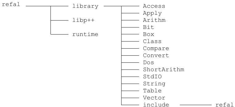
Рис. 2. Структура RSL
